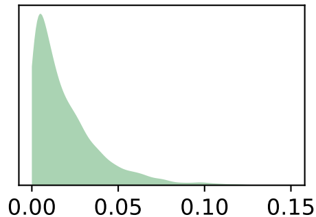
2_section_noise_d13c
