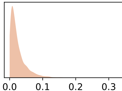
1_section_noise_d13c
