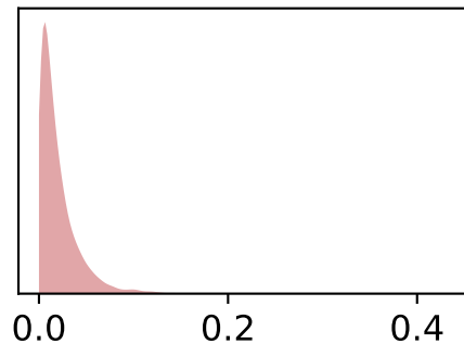
3_section_noise_d13c
