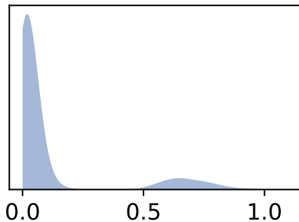
0_section_noise_d13c
