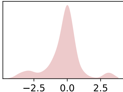
3_section_offset_d13c
