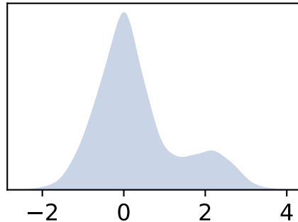
0_section_offset_d13c
