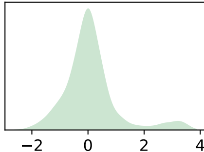
2_section_offset_d13c
