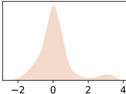
1_section_offset_d13c
