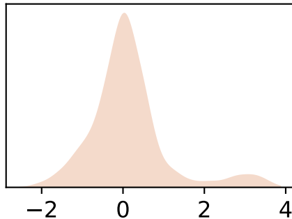
1_section_offset_d13c
