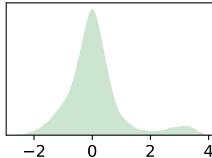
2_section_offset_d13c
