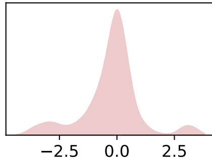
3_section_offset_d13c
