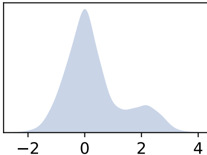
0_section_offset_d13c
