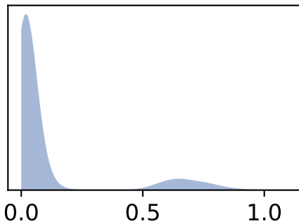
0_section_noise_d13c
