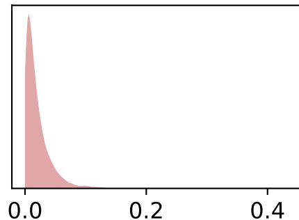
3_section_noise_d13c
