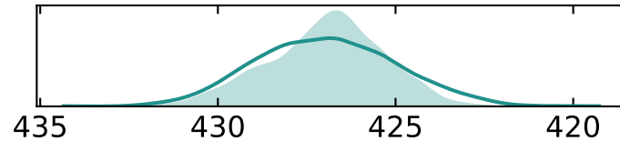
Detrital 1
