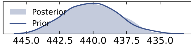
Detrital 0
